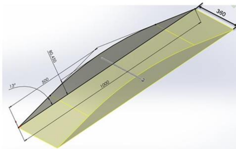
Şekil 3 Köprü ölçüleri
