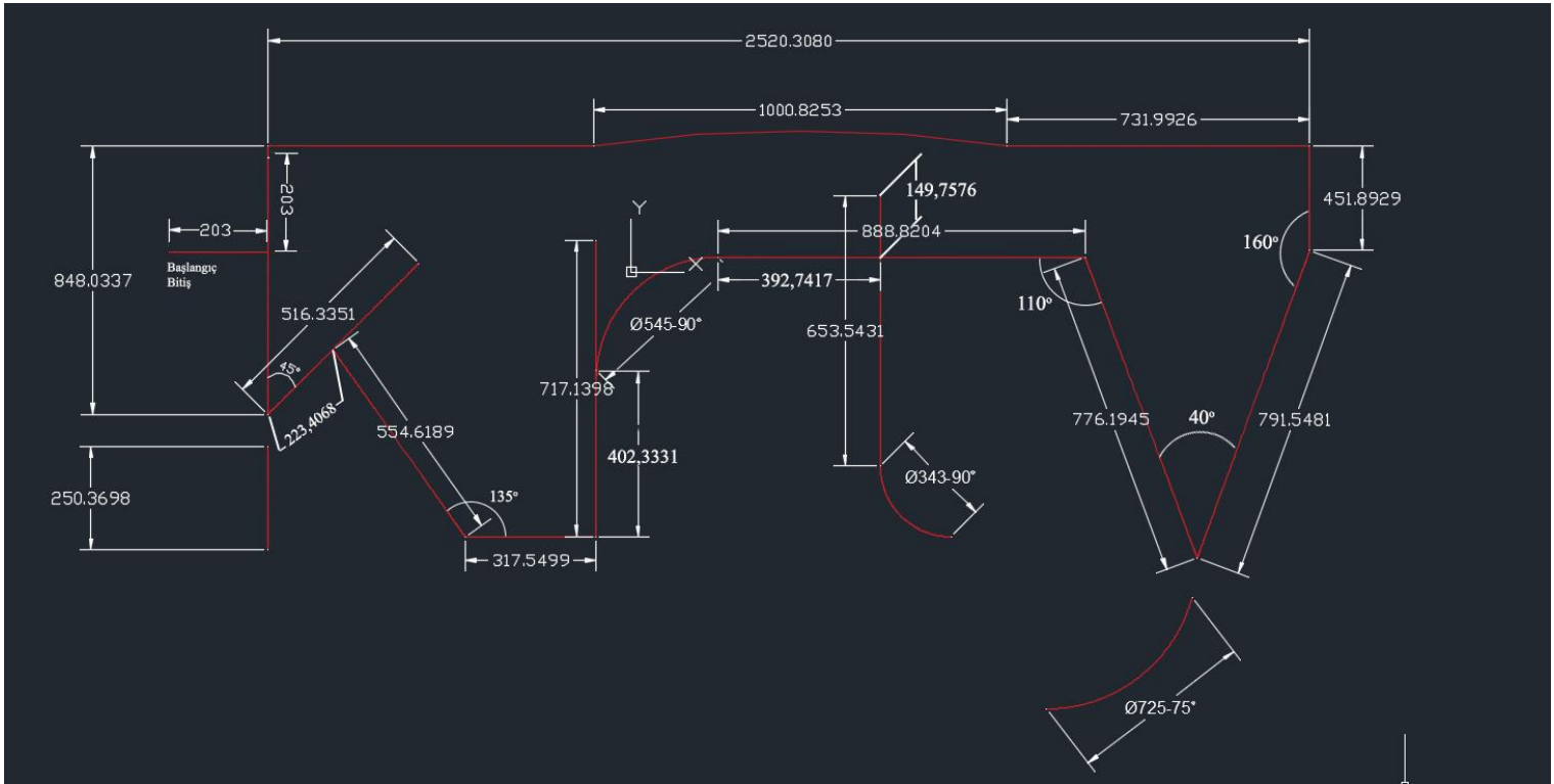
Şekil 2. Pist ölçüleri
